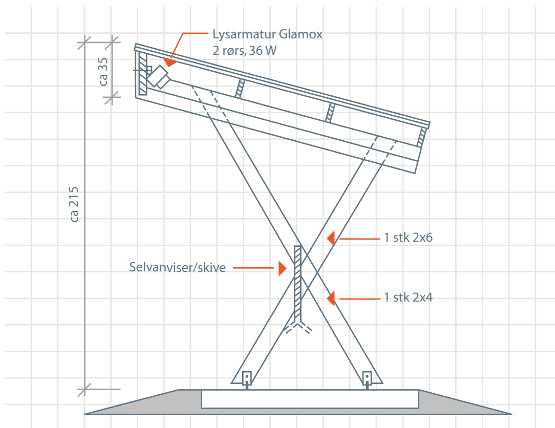
Skisse ovenfor viser eksempel på denne løsningen som er brukt i Valdres Skisenter i Skrautvål.
