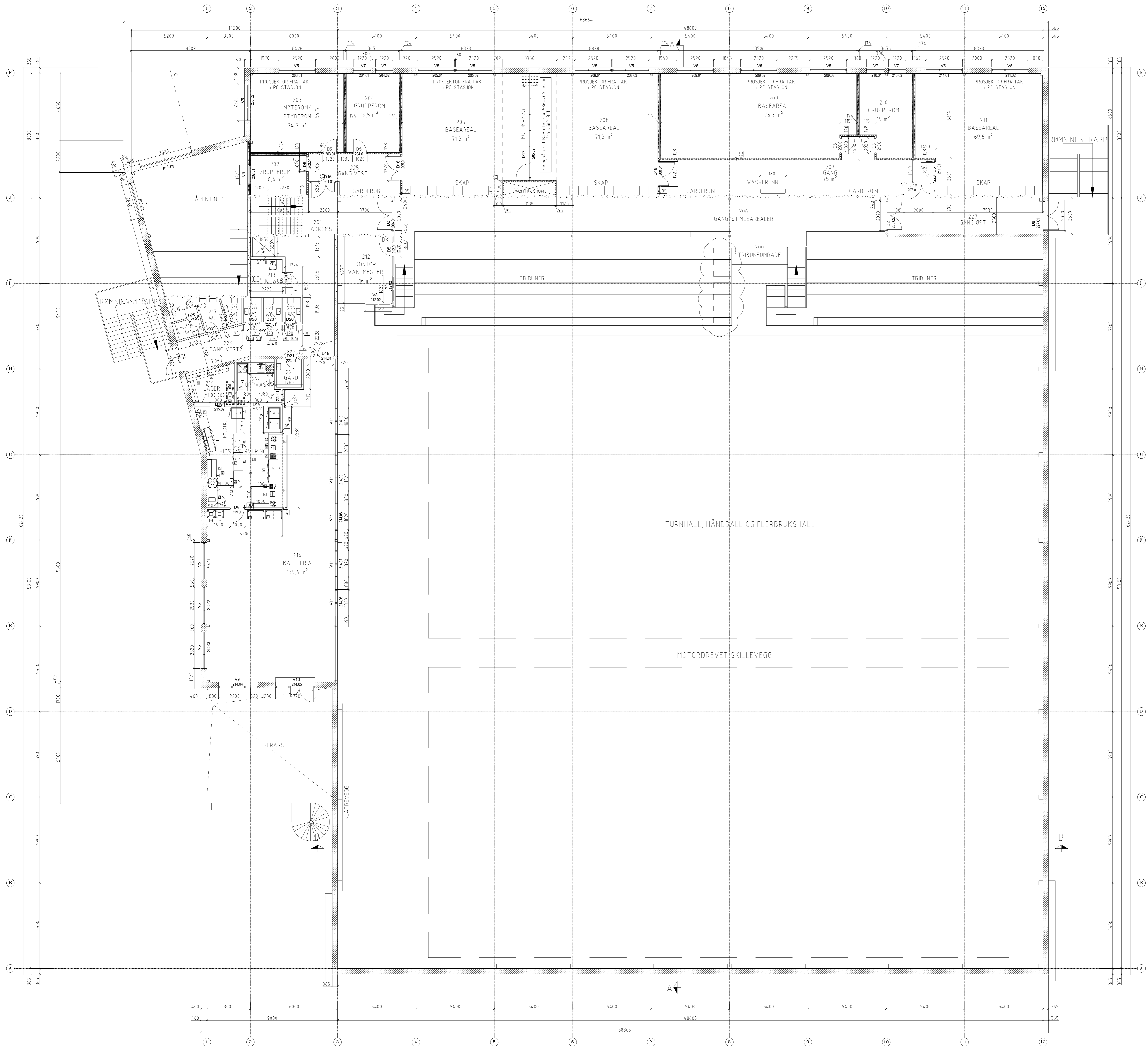
Plan 2.etg.
