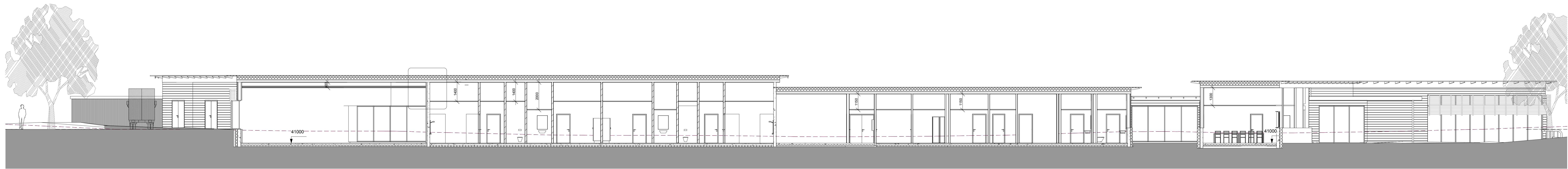
Snitt A-A 1-100 1 : 100
