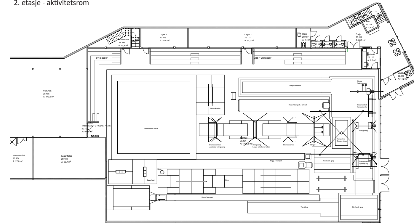
2. etasje - aktivitetsrom
